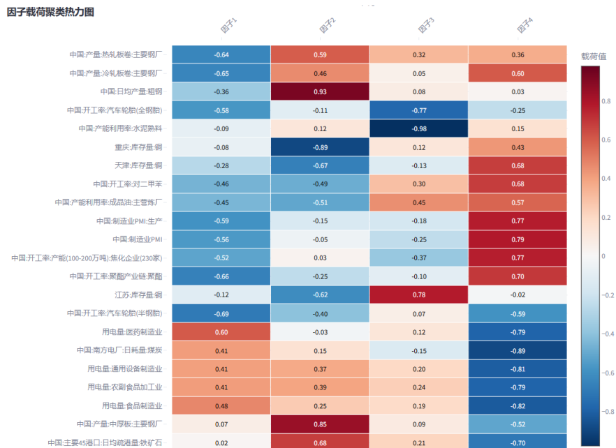
图 4.3.3 模型分析-因子载荷聚类热力图（经典 DFM 结果）
