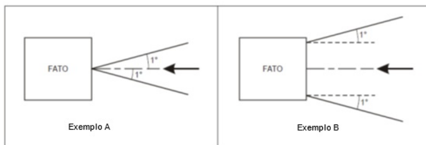
Figura 155.345-1 - Divergência do setor "trajetória correta"
