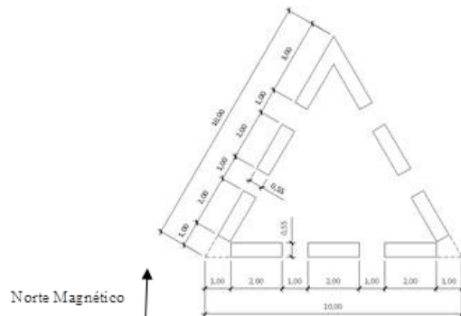
Figura 155.319-1 - Sinalização horizontal de ponto de visada de heliponto
