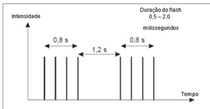
Figura 155.339-1 - Características do flash do Farol de Heliponto
