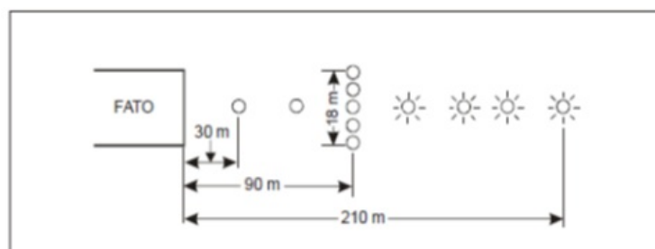
Figura 155.341-1 - Sistema de luzes de aproximação
