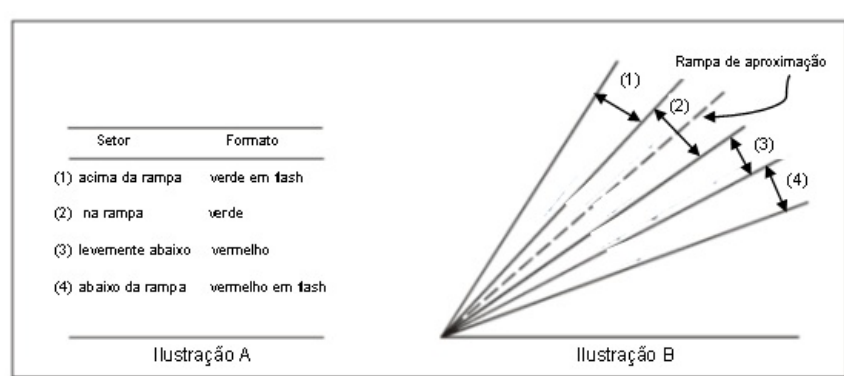
Figura 155.347-1 - Formato do sinal HAPI
