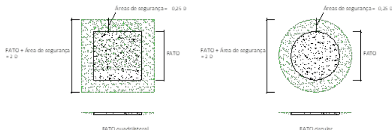
Figura 155.209-1 - FATO e área de segurança associada.
