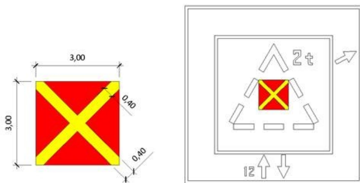
a) Dimensões da sinalização horizontal de interdição de FATO
