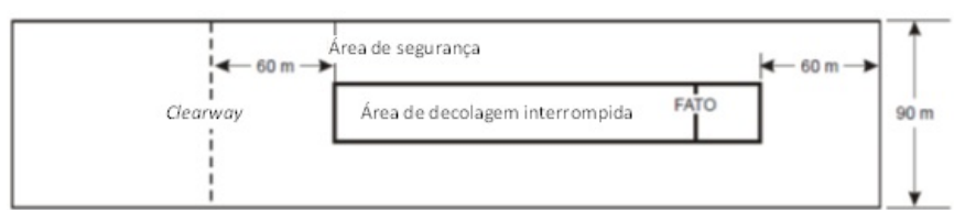
Figura 155.209-3 - Área de segurança para FATO com operação por instrumento
