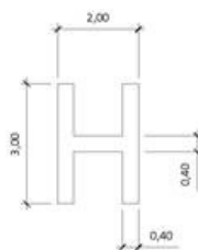
Figura 155.303-1 - Sinalização horizontal de identificação de heliponto.
