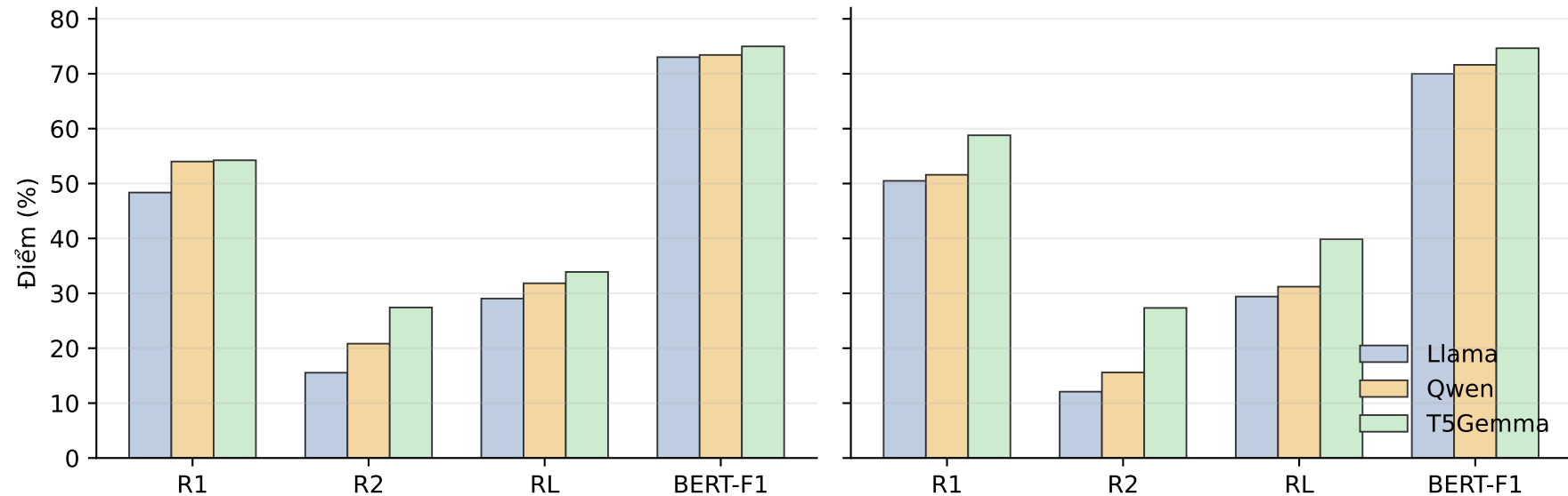
WikiLingua
