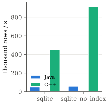
Insert, N = 100k
