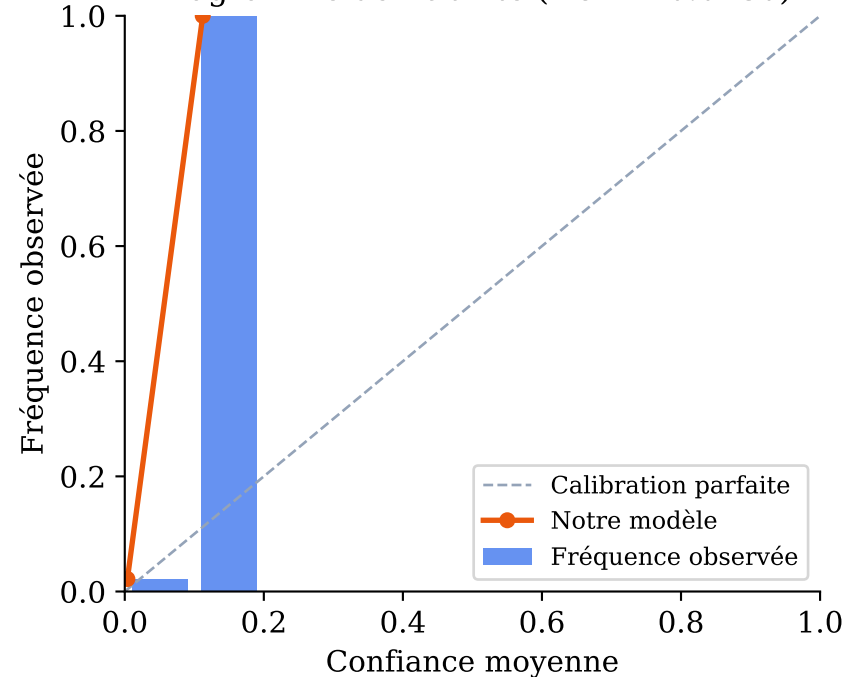
Diagramme de fiabilité (ECE = 0.0180)
