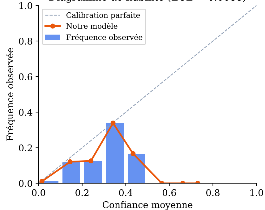
Diagramme de fiabilité (ECE = 0.0088)
