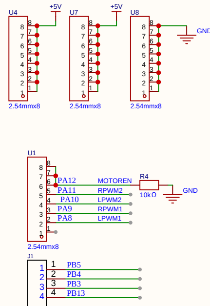
电机控制 供电引出
