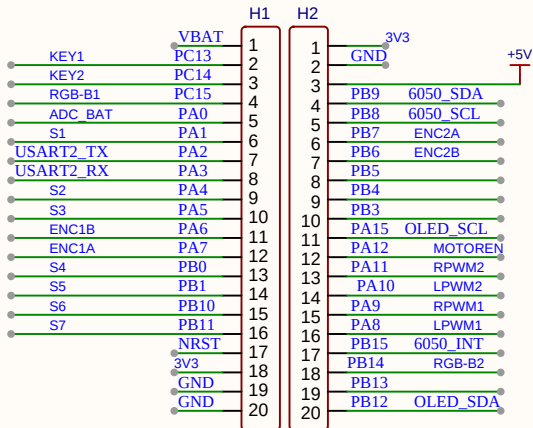
主控部分 单片机模块内部有5V降至3.3V
