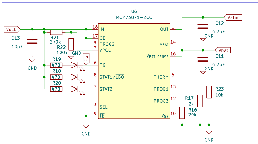
Chargeur de batterie intelligent
