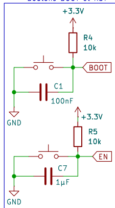
Boutons BOOT et RST
