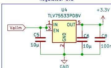
Régulateur 3v3
