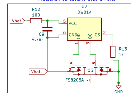
Protection de batterie avec un BMS
