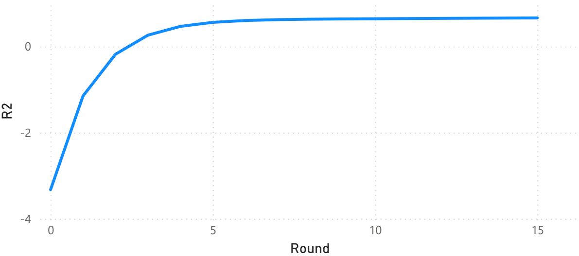
Convergence de l'apprentissage federe (R² par round)
