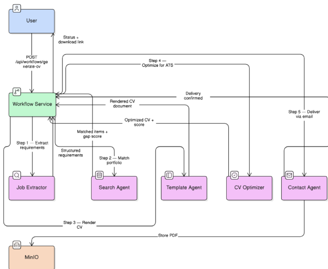
FIGURE 4.22 – Pipeline de génération de CV — De l’offre d’emploi à l’envoi par email
