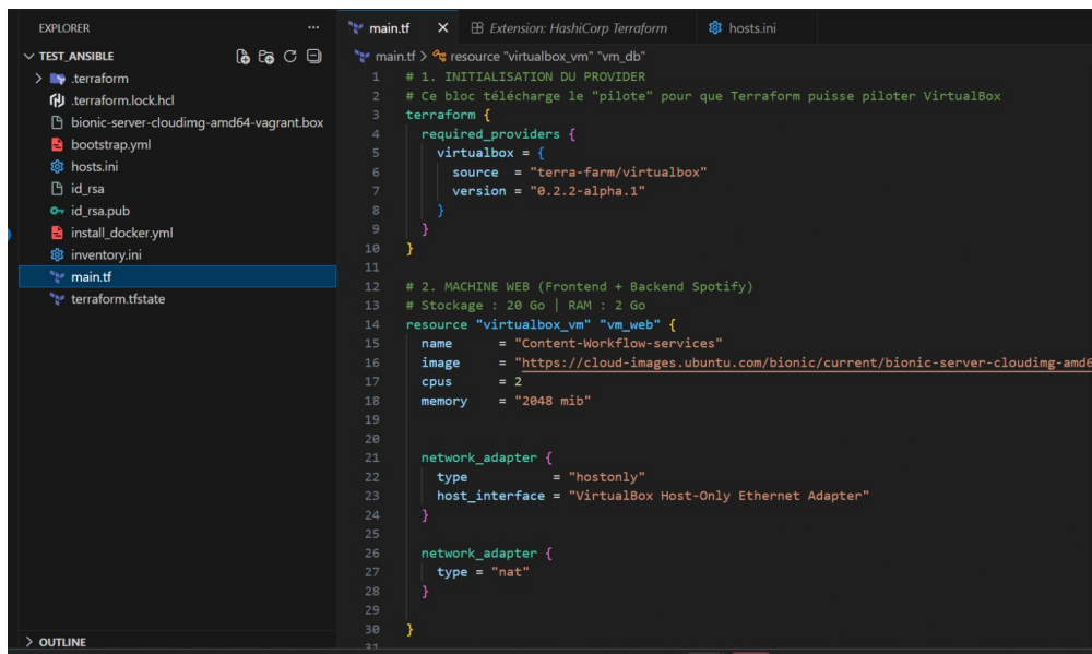
FIGURE 4.2 – Script Terraform — Définition des ressources VMs
