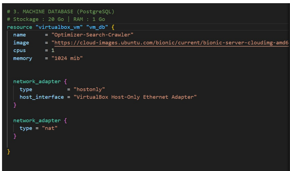
FIGURE 4.3 – Script Terraform — Configuration réseau et déploiement
