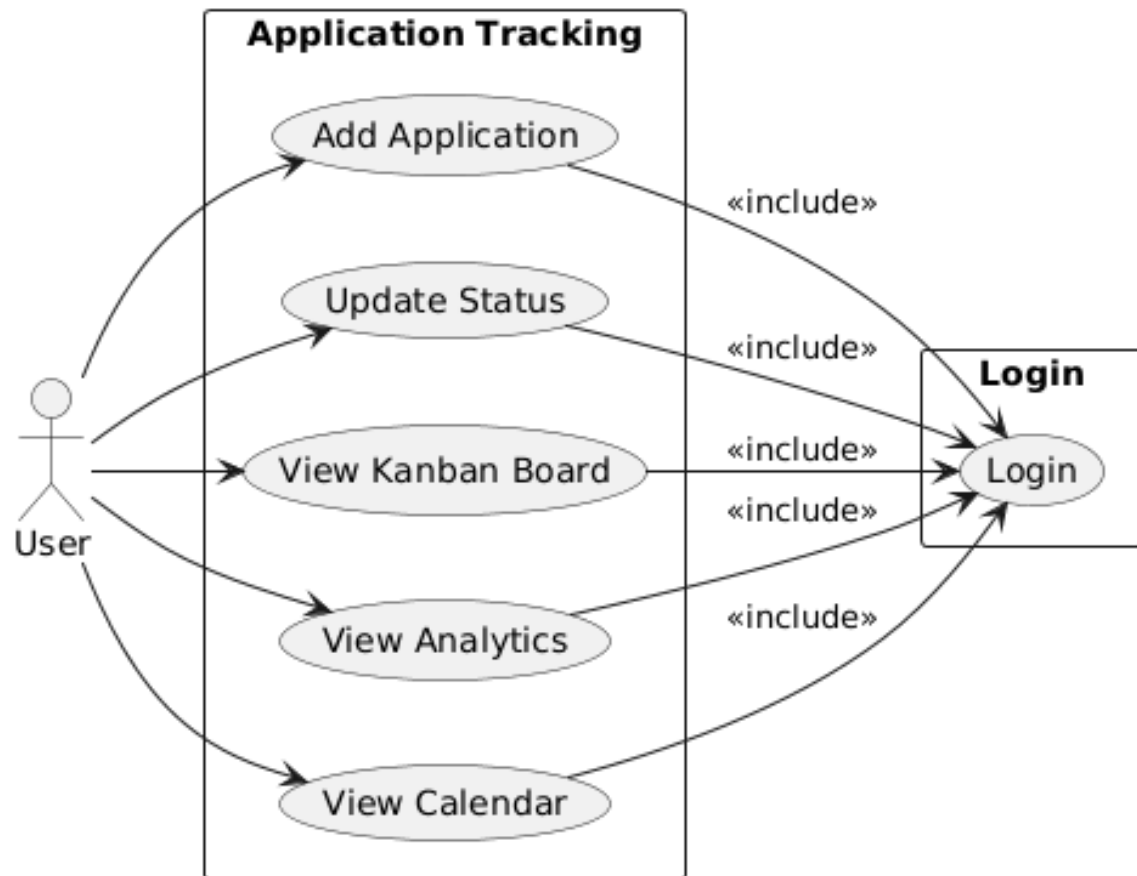
FIGURE 3.4 – Cas d'utilisation — Suivi des candidatures
