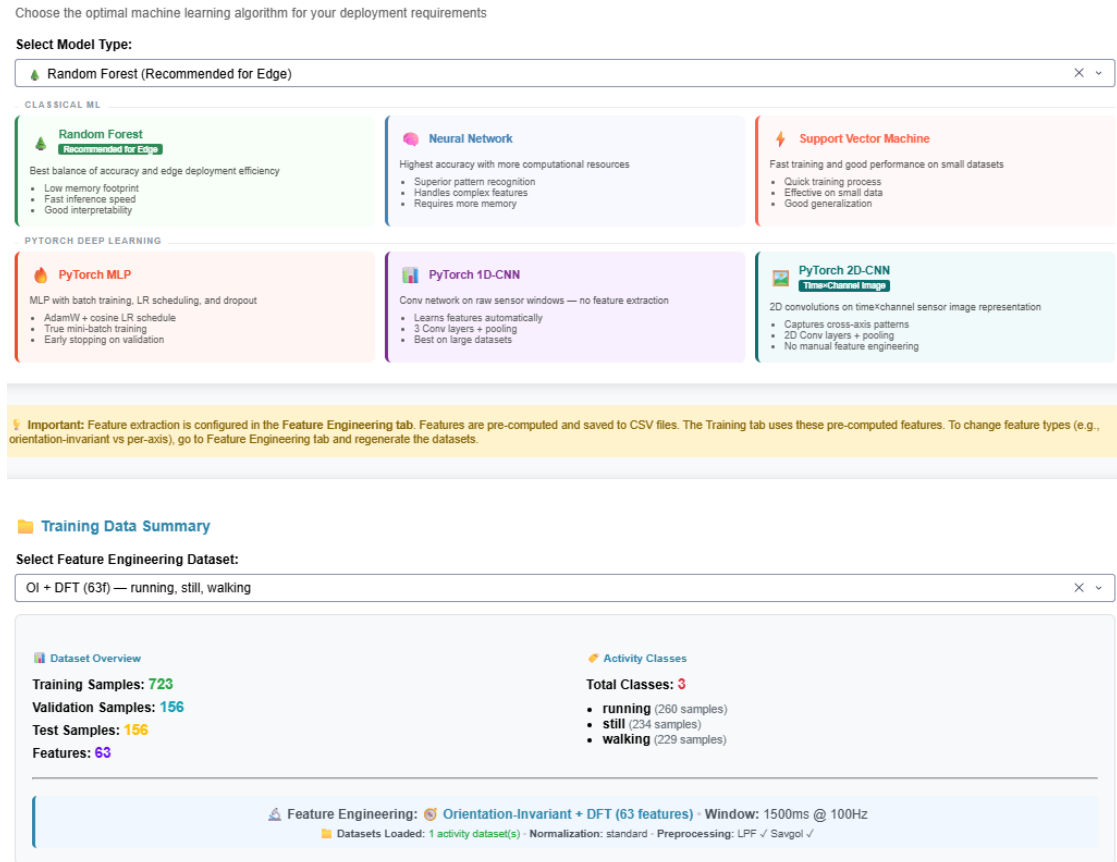
Hình 4.4 Giao diện cấu hình huấn luyện mô hình. Người dùng chọn thuật toán, cấu hình tối ưu hóa siêu tham số với GridSearchCV, chiến lược cân bằng lớp, và theo dõi tiến trình huấn luyện thời gian thực.
