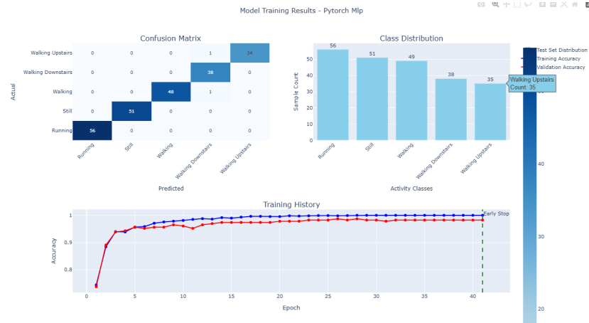
Hình 5.1 Ma trận nhầm lẫn — PyTorch MLP, bài toán 5 lớp (tập kiểm tra 229 mẫu). Các lỗi phân loại tập trung ở nhóm hoạt động đi bộ: 1 mẫu walking bị nhầm thành walking_downstairs (hàng walking, cột W.Down).
