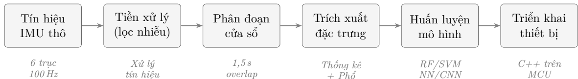
Hình 1.1 Quy trình HAR dựa trên IMU: từ thu thập tín hiệu thô đến triển khai trên vi điều khiển
