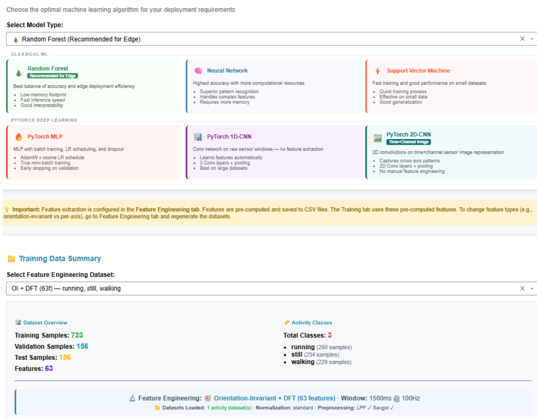
Hình 4.4: Giao diện cấu hình huấn luyện mô hình. Người dùng chọn thuật toán, cấu hình tối ưu hóa siêu tham số với GridSearchCV, chiến lược cân bằng lớp, và theo dõi tiến trình huấn luyện thời gian thực.
