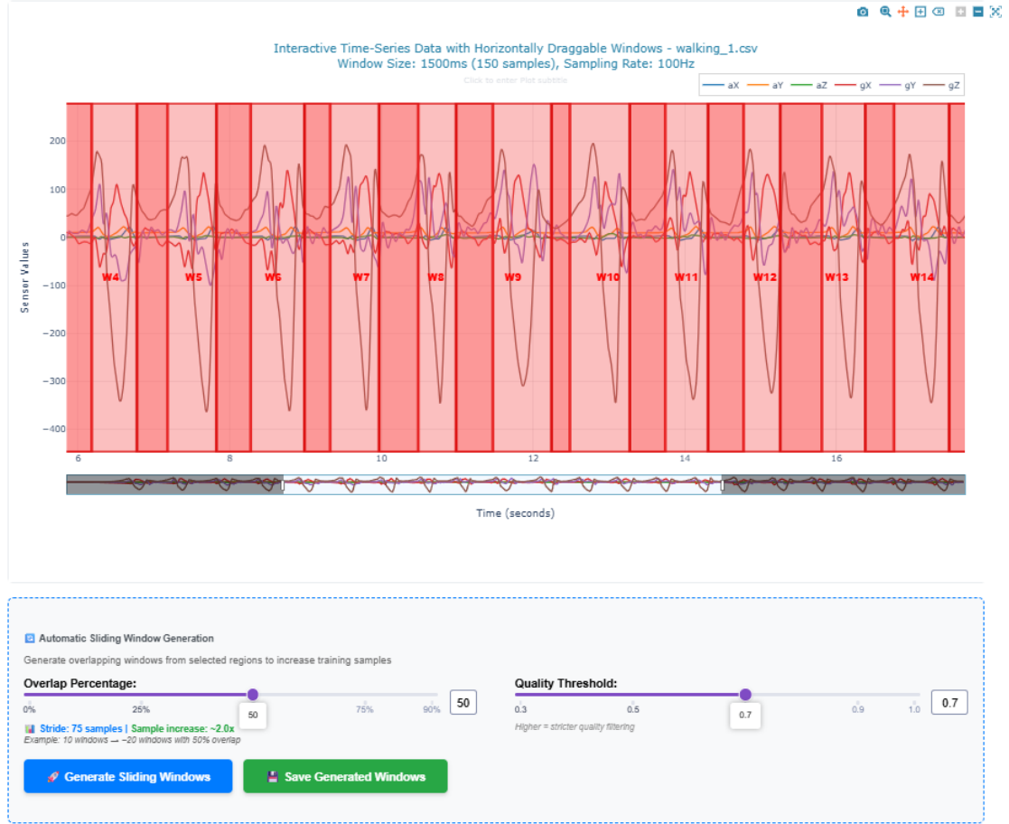
Hình 4.2: Giao diện cửa sổ kéo thả tương tác. Người dùng kéo thả trực tiếp trên biểu đồ tín hiệu để xác định các đoạn hoạt động đại diện. Cửa sổ trượt tự động sinh các mẫu huấn luyện từ các đoạn đã chọn, kết hợp giữa kiểm soát thủ công và tự động hóa.
