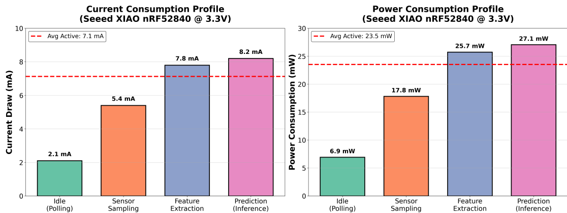
Hình 4.4.2: Hồ Sơ Tiêu Thụ Điện Năng Trong Suy Luận (Neural Network, Chế Độ Accuracy)
