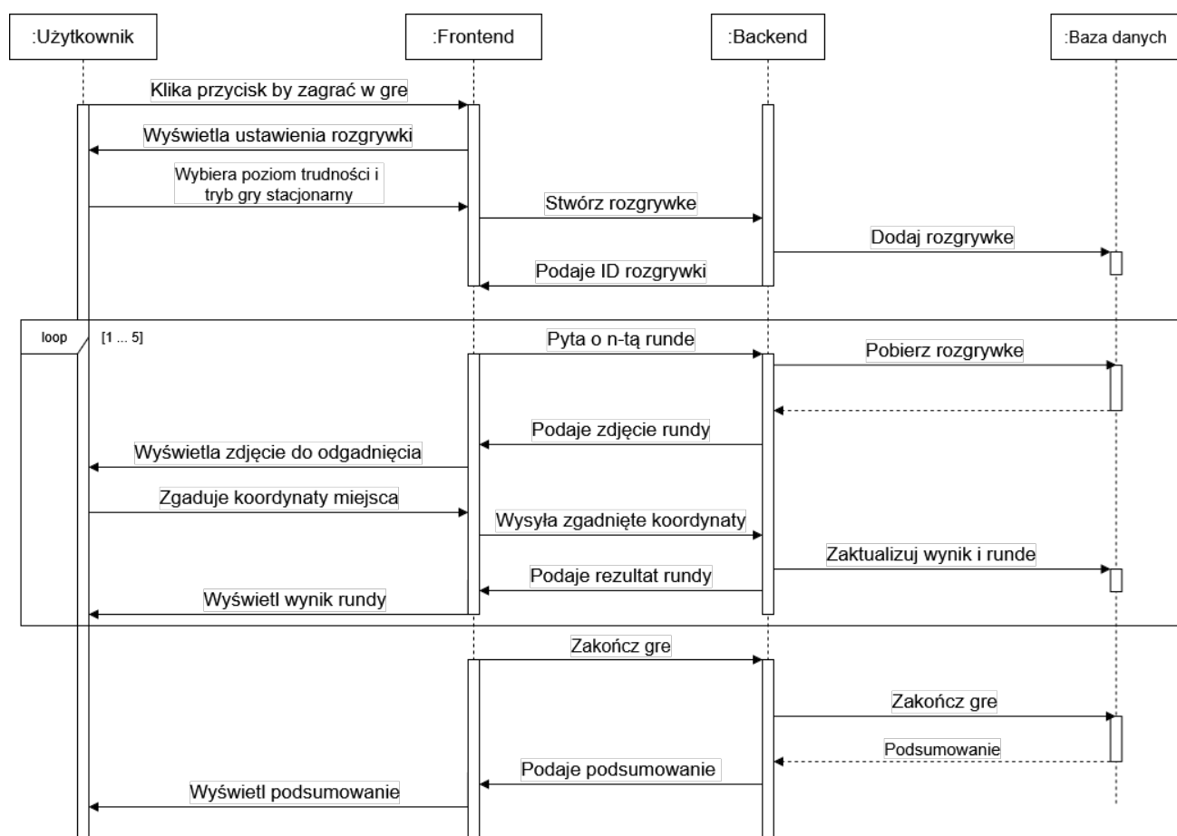
Rysunek 7.4: Diagram sekwencji przedstawiający przebieg rozgrywki w aplikacji UniGuesser
