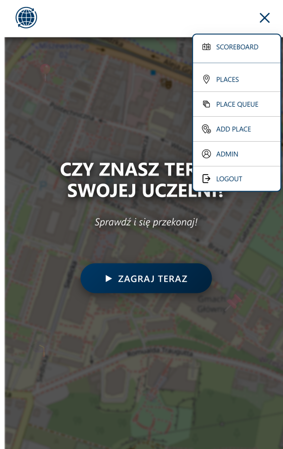
Rysunek 8.2: Hamburger menu w widoku mobilnym aplikacji UniGuesser
