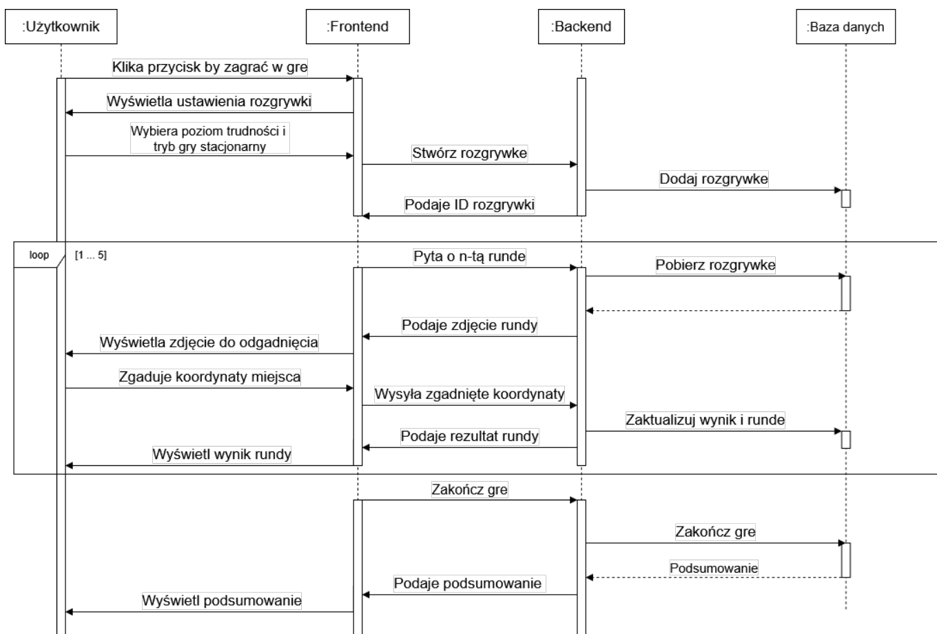
Rysunek 7.4: Diagram sekwencji przedstawiający przebieg rozgrywki w aplikacji UniGuesser
