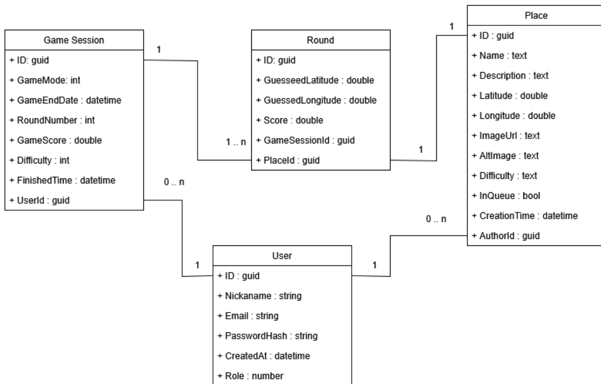
Rysunek 6.4: Diagram ERD dla bazy danych aplikacji UniGuesser
