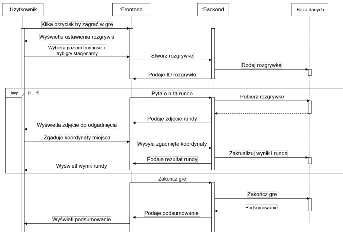
Rysunek 6.6: Diagram sekwencji przedstawiający przebieg rozgrywki w aplikacji UniGuesser
