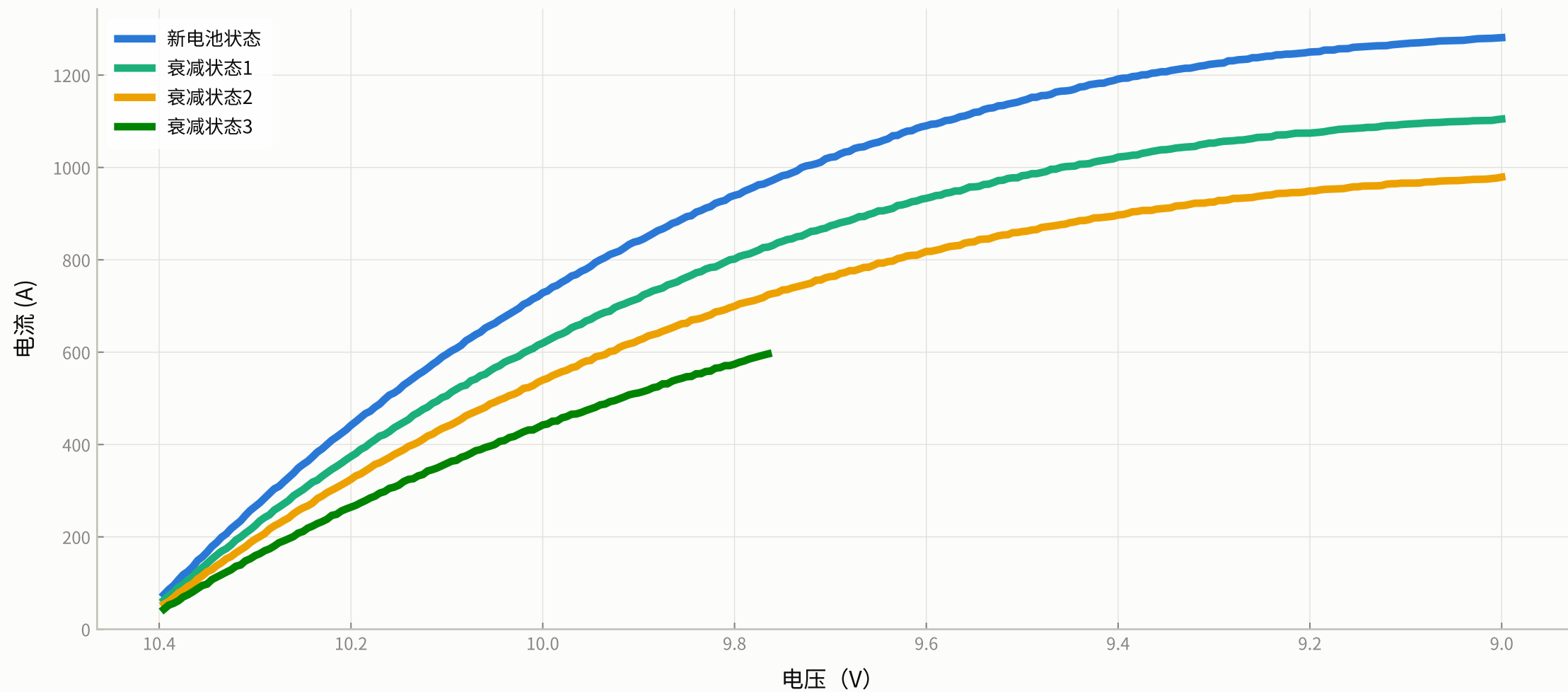
电池状态随电压变化曲线
