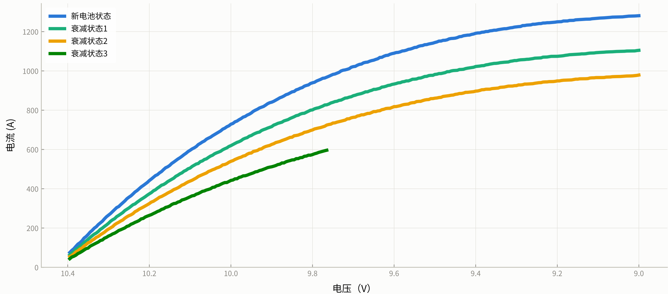
电池状态随电压变化曲线
