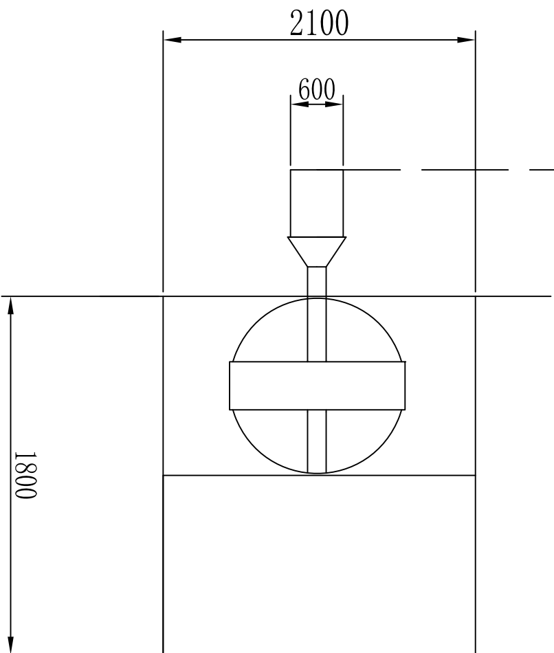
俯视图
