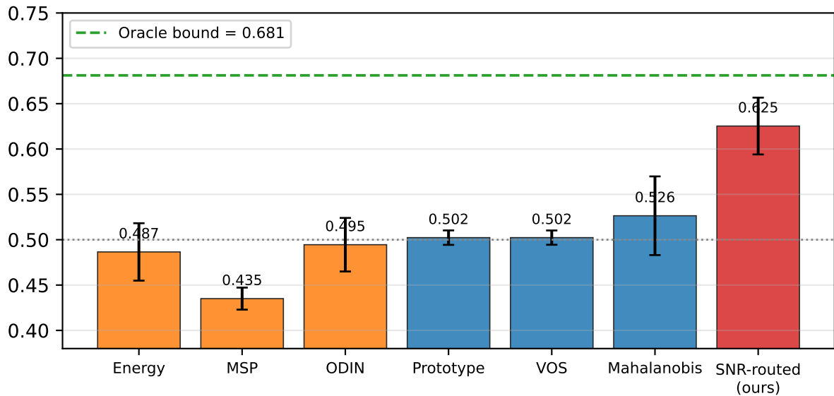
Weighted-avg OOD AUROC
