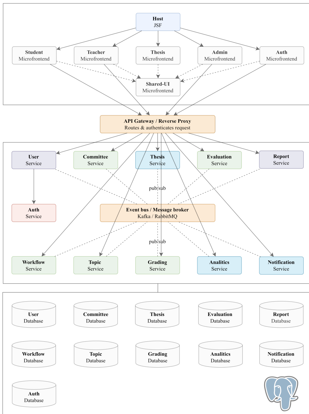
Зураг 5.4. Системийн бүрэн архитектурын нэгдсэн бүдүүвч
