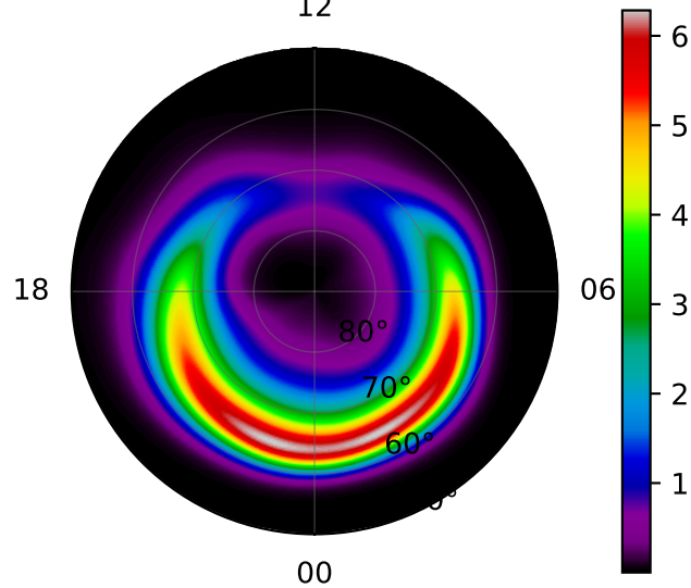
Model Q ( \text{mW m}^{-2} )
