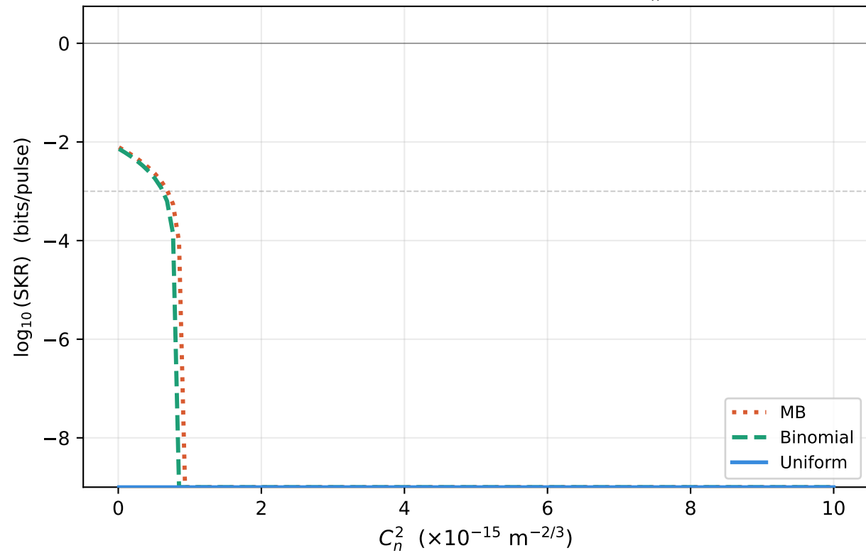
(d) SKR vs Turbulence Strength C_n^2
