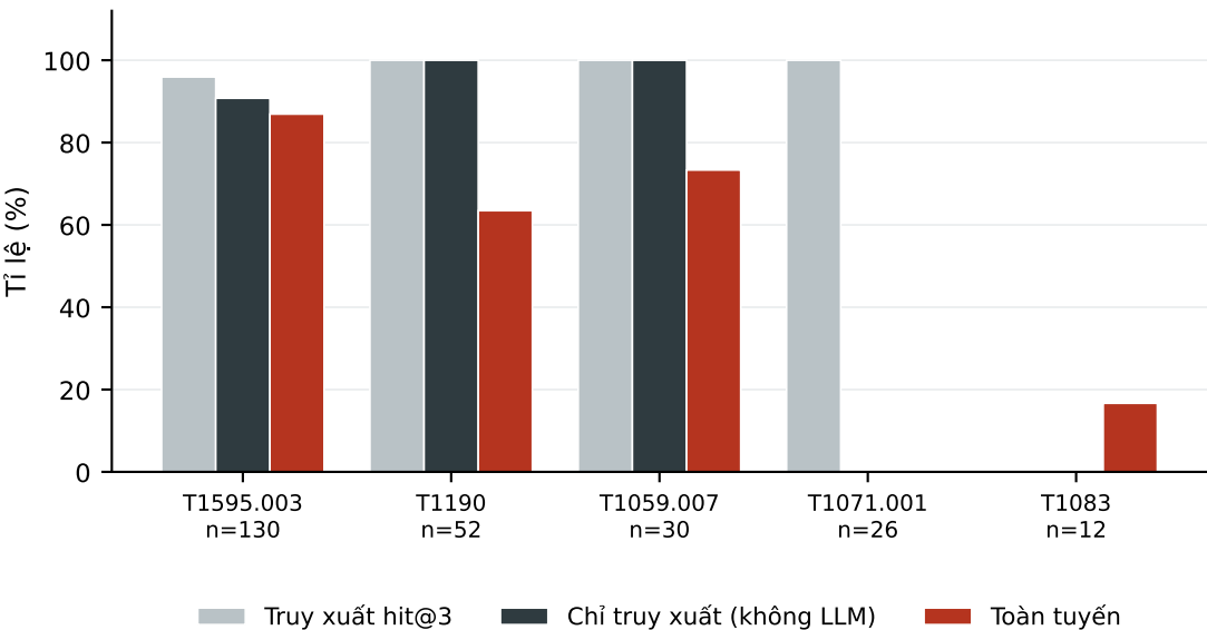
Quy kết theo từng kỹ thuật, đặt cạnh trần truy xuất
