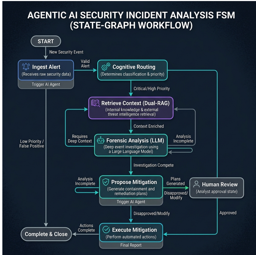
Hình 2.2: Quy trình phân tích sự cố của hệ thống AI Tác tử dựa trên mô hình Đồ thị Trạng thái (FSM).
