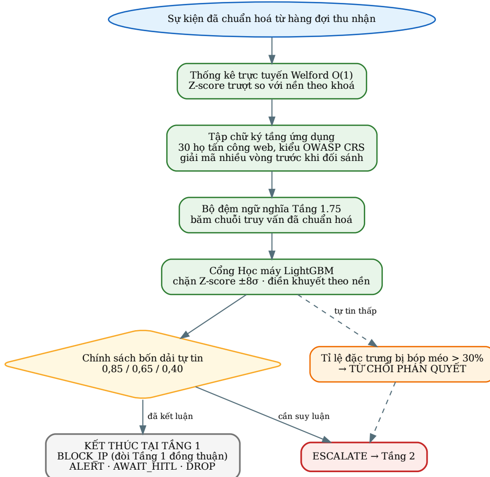
Hình 2. Tầng 1 phóng to. Chỉ nhánh ESCALATE đi tới Tầng 2; mọi phán quyết khác kết thúc tại đây, và đó chính là thứ Chương 4 tính là xả tải. (Nguồn: Tác giả)
