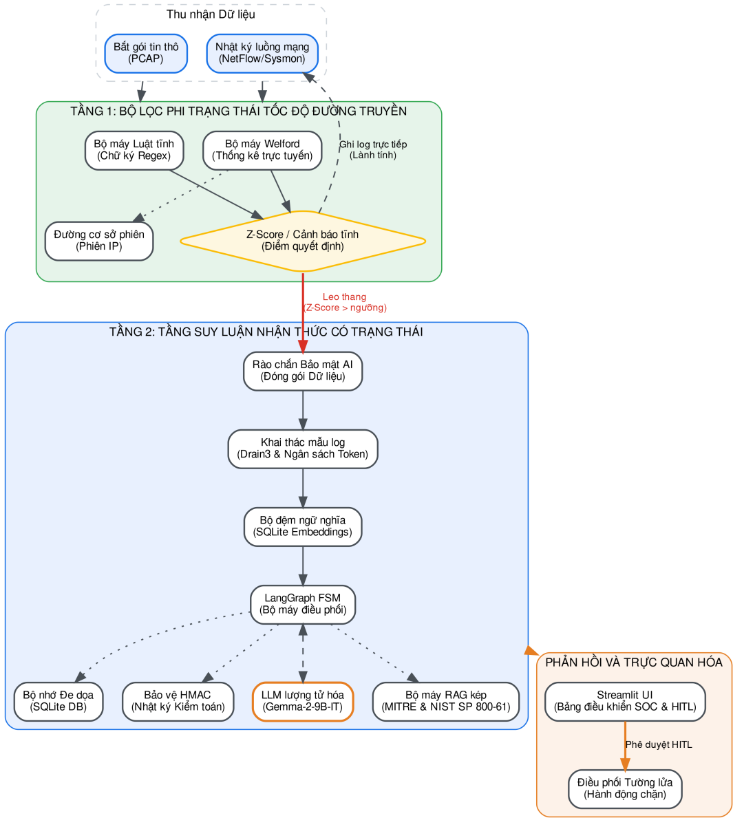
Hình 4. Sơ đồ kiến trúc tổng thể của hệ thống SENTINEL, minh họa luồng dữ liệu hai tầng và các thành phần cấu trúc. (Nguồn: Tác giả)
