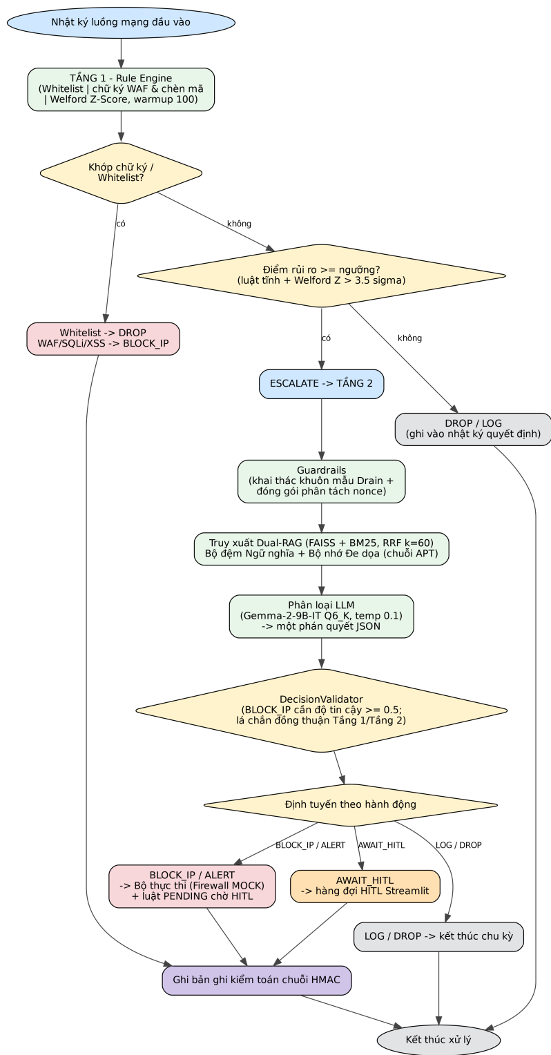
Hình 5. Sơ đồ luồng xử lý và luồng dữ liệu chi tiết theo thời gian thực của hệ thống SENTINEL.
