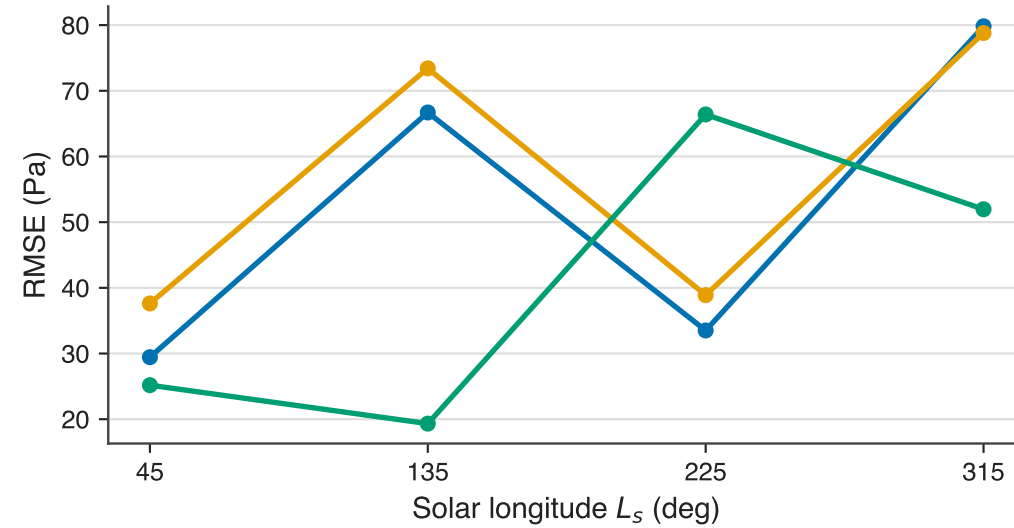
Surface CO2 frost
