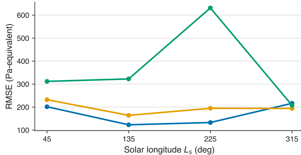
Surface CO2 frost
