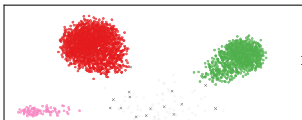
Layer 17 — modules (7)
