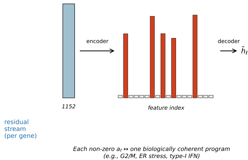
(B) Sparse autoencoder
