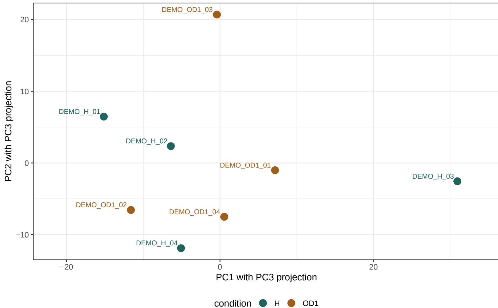
3D PCA projection – lncRNA OD1 vs H
