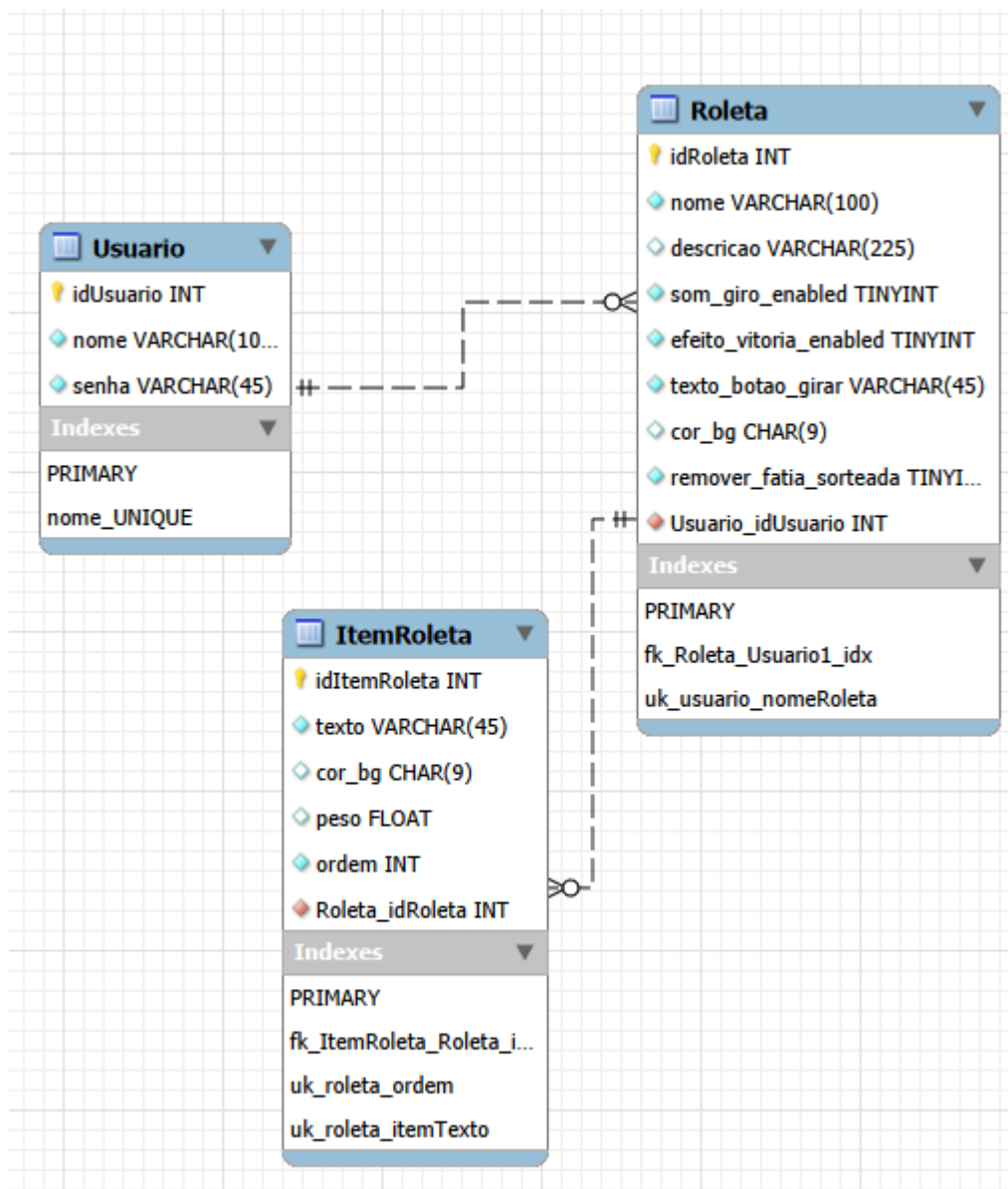
Figura 1 — Modelo lógico (tabelas e integridade referencial).
