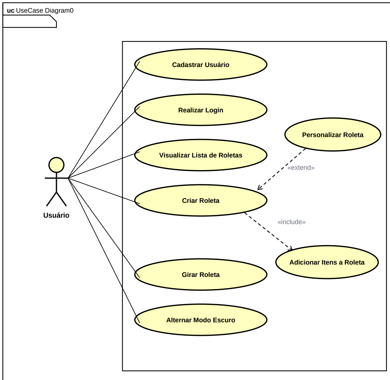
Figura 1 — Diagrama de casos de uso (UML) do Sistema de Roletas Personalizadas.
