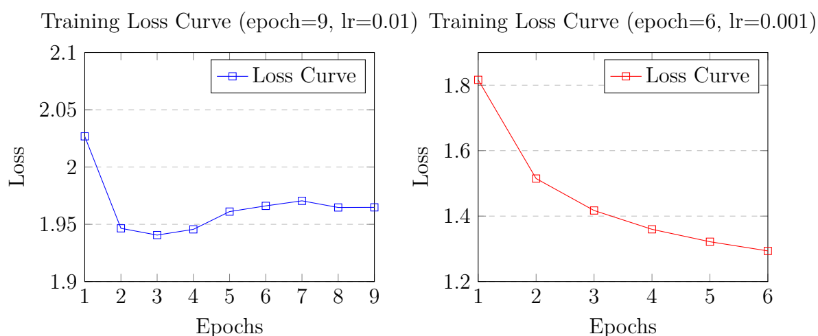
图 2: 在不同 epoch 和学习率下的训练损失曲线：这些配置并非最优解
