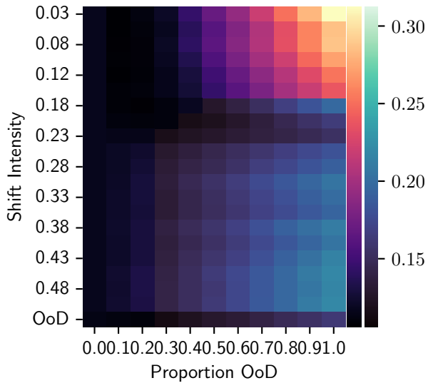
Dataset = Polyp
