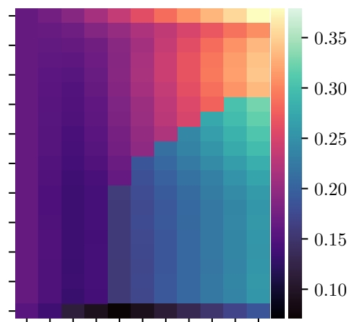
Dataset = NICO
