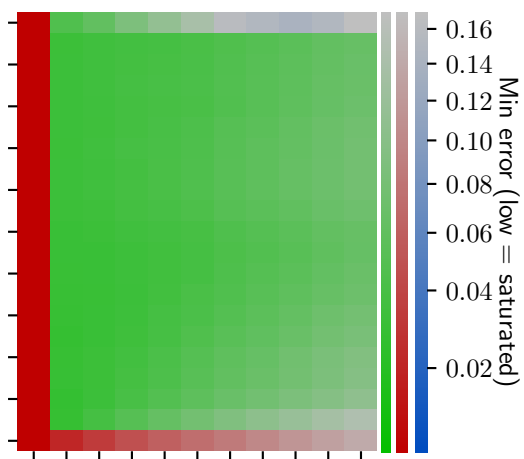
Dataset = NICO
