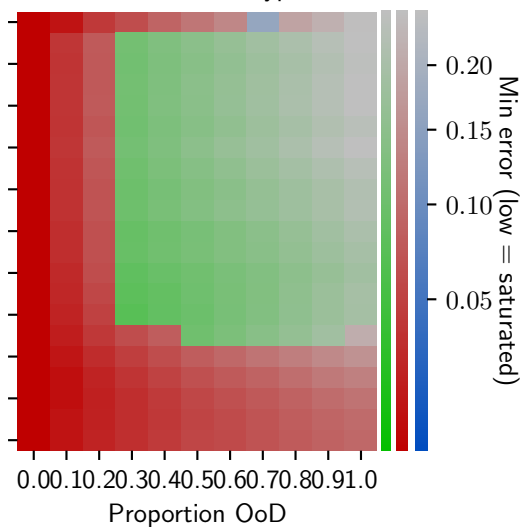
Dataset = Polyp
