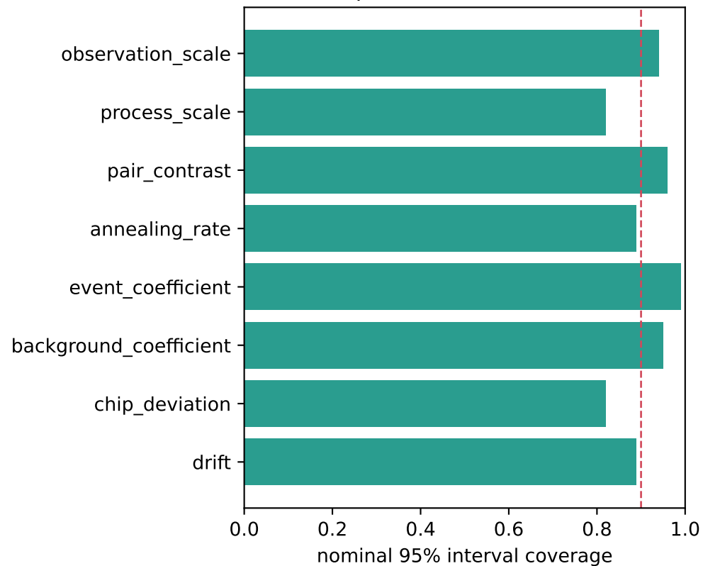
V2 Laplace interval calibration
