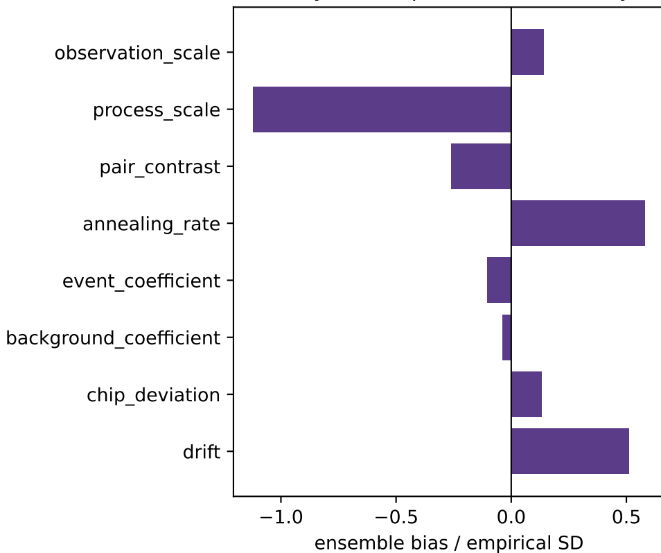
V2 synthetic parameter recovery
