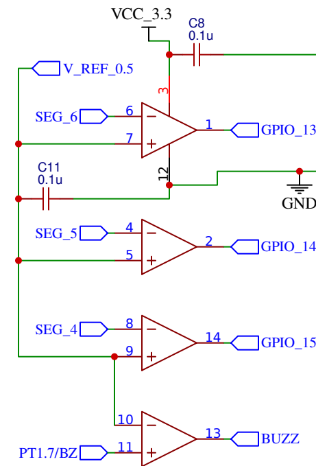
U4 - LM339LVPWR
