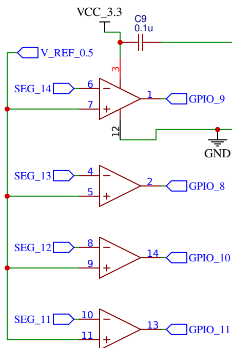
U5 - LM339LVPWR
