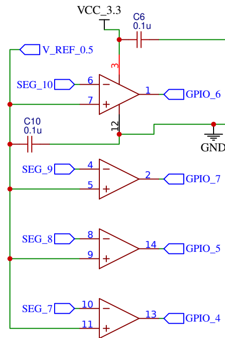
U3 - LM339LVPWR
