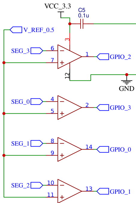
U1 - LM339LVPWR
