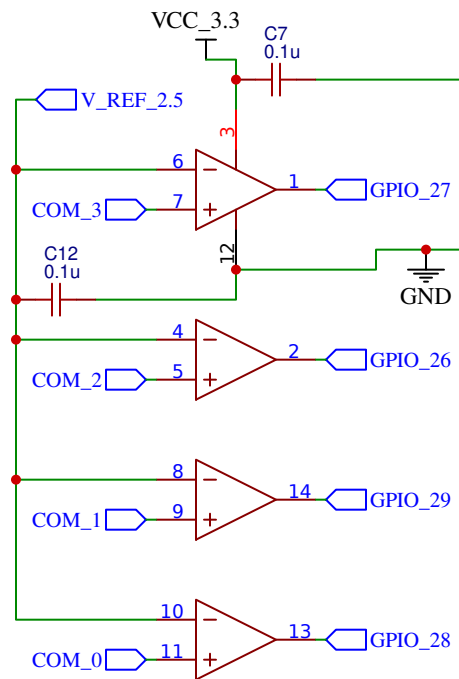
U2 - LM339LVPWR
