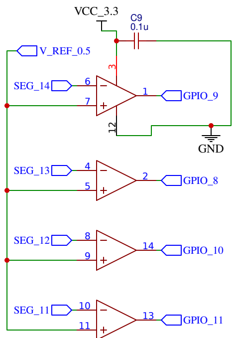
U5 - LM339LVPWR
