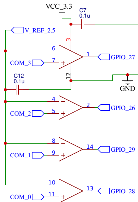
U2 - LM339LVPWR
