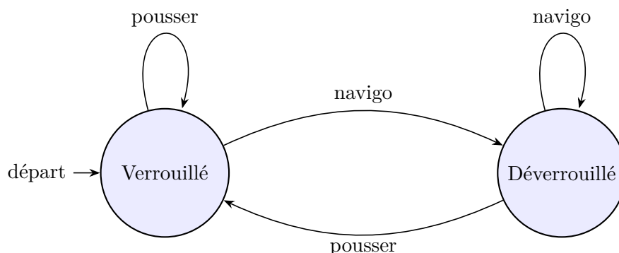
Figure 2 – Automate d'un tourniquet.
