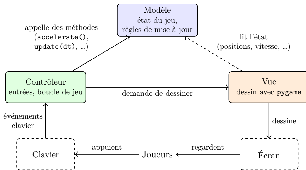
Figure 1 – Les trois parties de l'architecture MVC et la façon dont elles communiquent. La flèche en pointillés signifie que la vue ne fait que lire le modèle.
