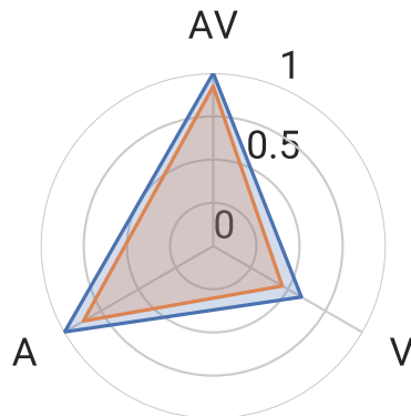
Equi-AV
