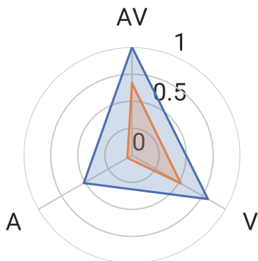
Gemini 1.5 Flash
