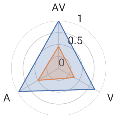
VideoLLaMA 2
