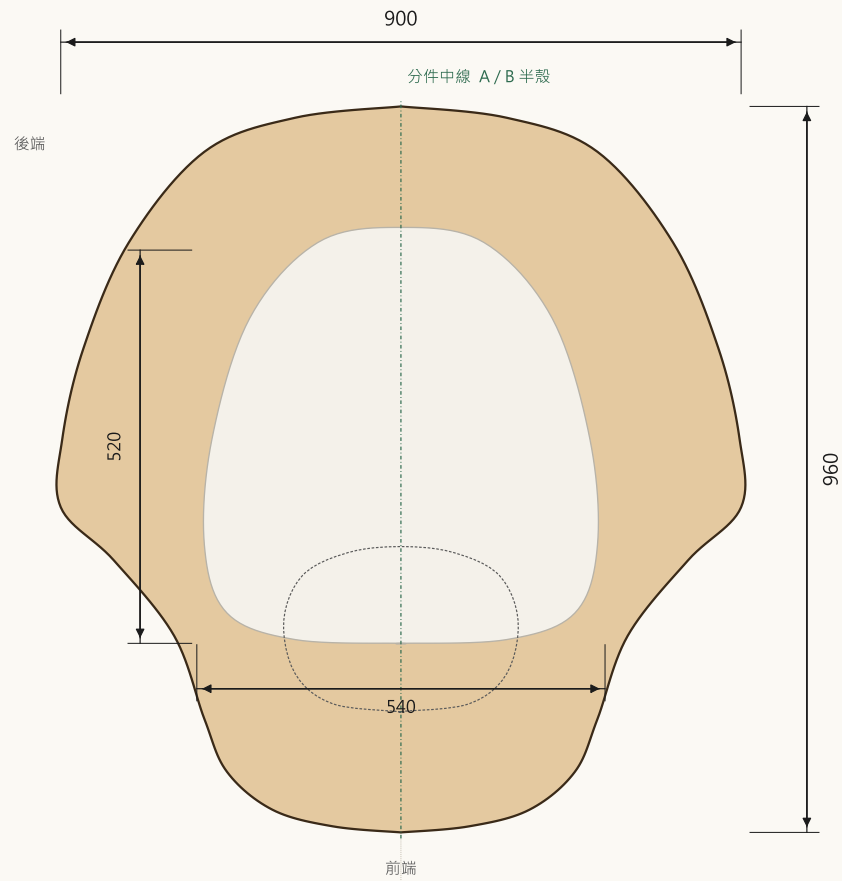
俯視圖 TOP
