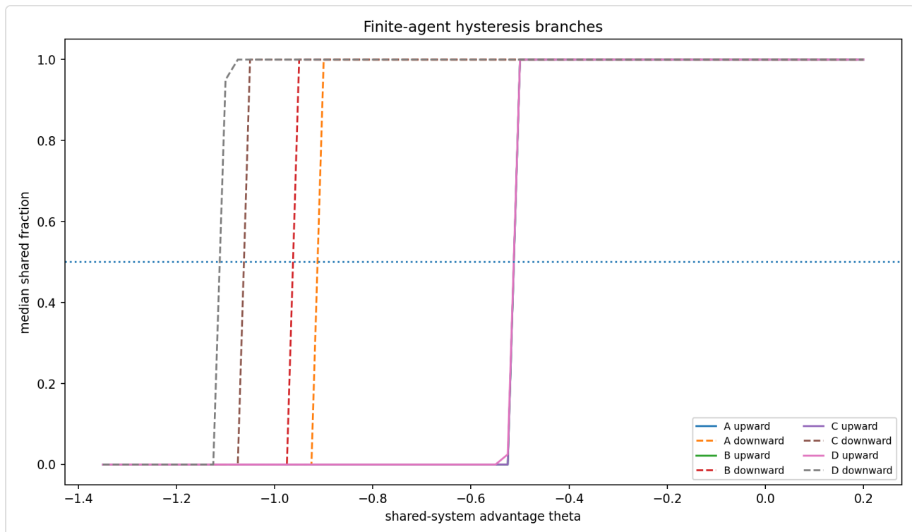
Figur 2.1 — Hysteresgrenar för ändliga agenter för de fyra avklingning \times spärr-cellerna. Alla celler delar en inträdeströskel; återgångströsklarna separerar.
