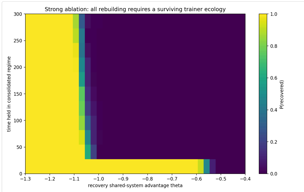
Figur 6.4 — Den fullt grindade ablationen. Under det namngivna tränar-livskraftighetsantagandet framträder en betingat nära-absorberande region.
