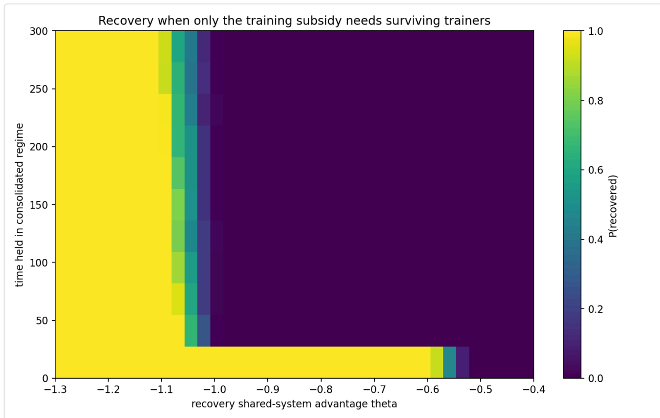
Figur 6.1 — Återhämtningssannolikhet över låsvaraktighet \times återhämtningstryck, fast återuppbyggnadseffektivitet.
