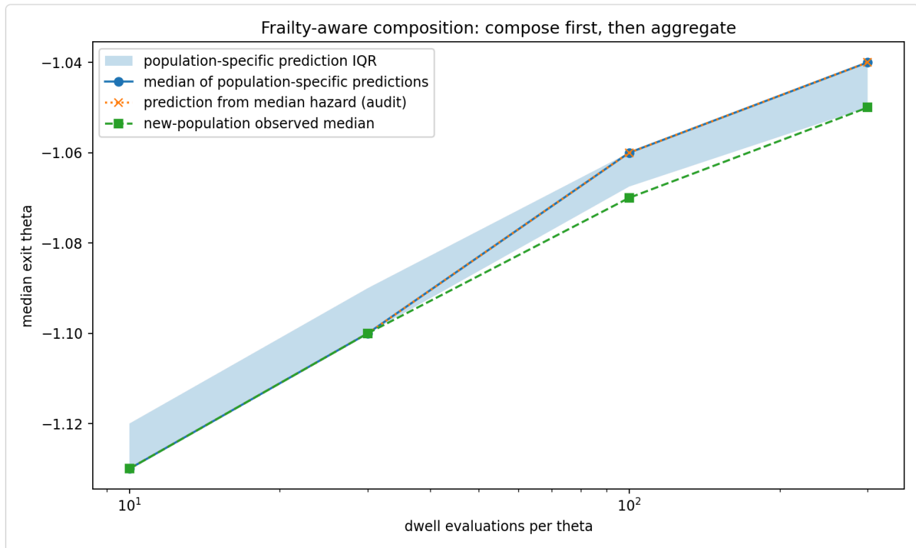
Figur 5.3 — Fasta- \theta -faror, uppmätta oberoende och sammansatta per population utan några anpassade uppehållsparametrar, mot observerade medianer på nya populationsdragningar.
