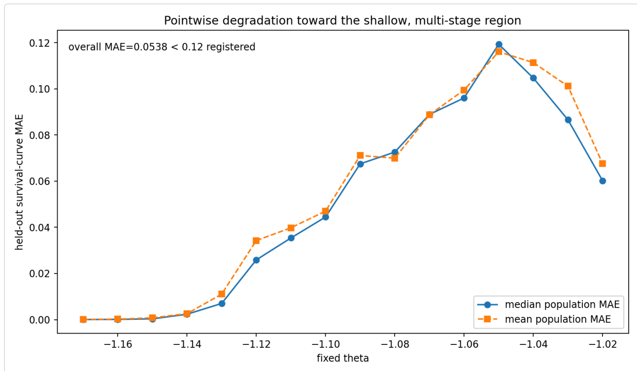
Figur 5.2 — Undanhållet överlevnadskurvfel för exponentialreduktionen över \theta -rutnätet, mot den registrerade gränsen för det övergripande medelvärde. Punktvis fel når en topp vid den grunda kanten, där flykt är flerstegs.
