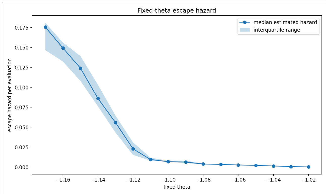
Figur 5.1 — Flyktfara per utvärdering vid fast \theta (median över populationer, interkvartilband). Faran spänner över tre storleksordningar över övergångsregionen.
