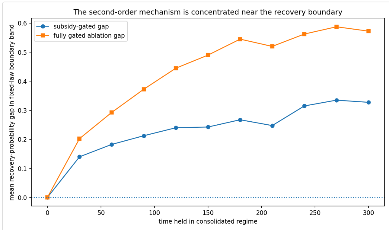
Figur 6.3 — Bandbetingat återhämtningsgap mot låsvaraktighet, för den subventionsgrindade lagen och den fullt grindade ablationen.
