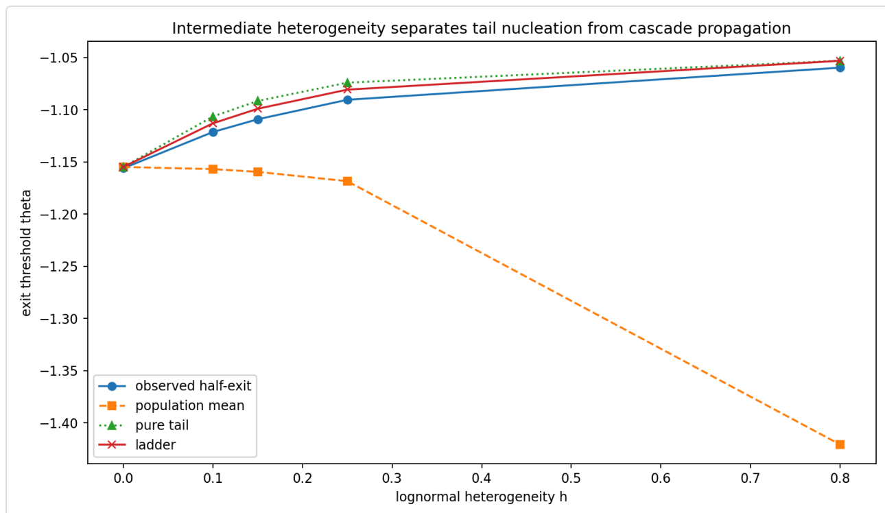
Figur 4.1 — Observerat halvtuttråde mot homogena, rena svans- och stegförutsägelser över heterogenitet. Stegen är mest distinkt från den rena svansen vid intermediärt h .
