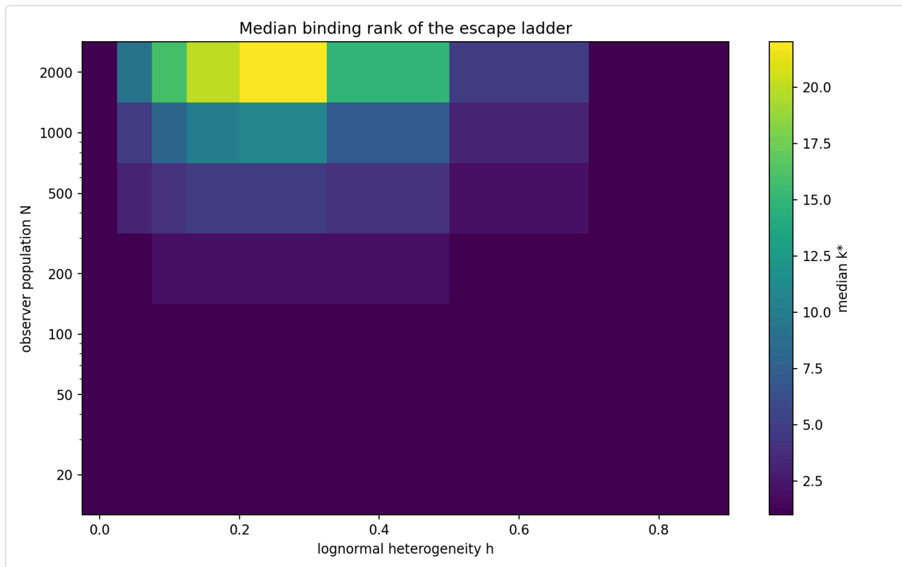
Figur 4.4 — Medianbindningsrang k^* över samma rutnät: den kvantitativa följeslagaren till faskartan.
