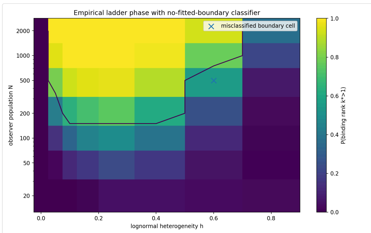
Figur 4.3 — Monte Carlo P(k^* > 1) över det frusna N \times h -rutnätet med den analytiska gränsen överlagrad; den enda felklassificerade cellen ligger på själva gränsen.
