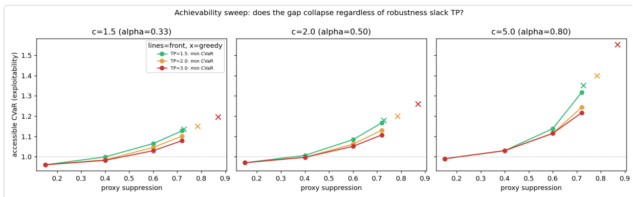
Figur 3. Uppnåelighetssvepning. Varje panel håller motståndarkoncentrationen c fast; kurvorna ger den minimalt uppnåeliga tillgängliga CVaR (en värdefunktion) mot proxy-undertryckning under tillåtelser för komplementär känslighet TP \in \{1.5, 2, 3\} , där kryss markerar den riskblinda proxy-giriga regulatören vid dess egen undertryckning. Golvet stiger monotont med undertryckning i
