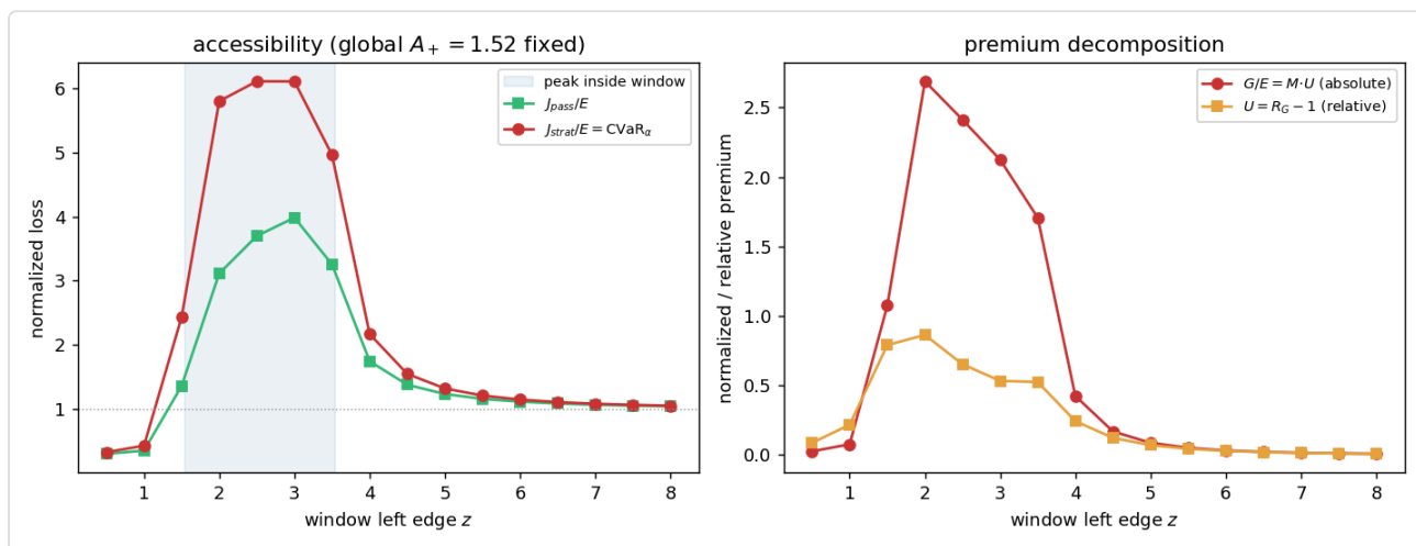
Figur 2. Vänster: passiv och strategisk förlust när ett nåbart fönster med fast bredd glider över frekvens, med den globala positiva log-arean A_+ hållen fast genomgående; realiserad förlust följer huruvida fönstret innehåller den förstärkta regionen, inte den konserverade totalen —
