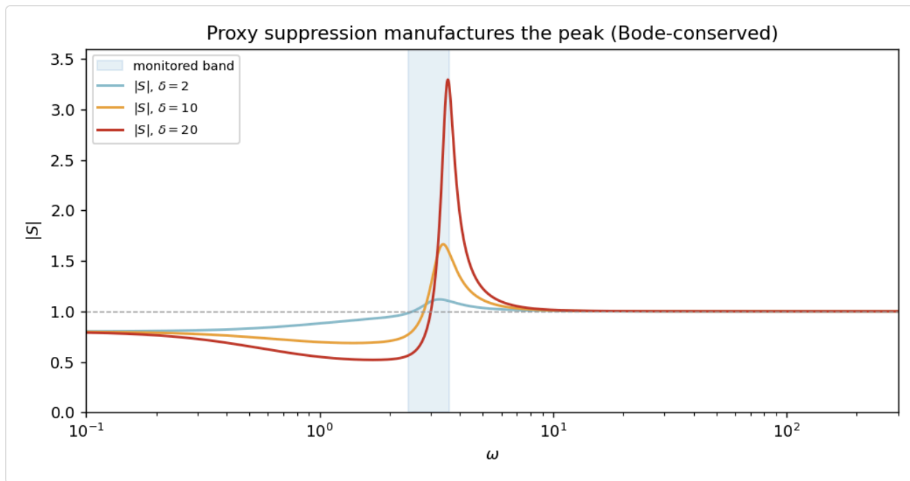
Figur 1. Övervakad-band-undertryckning framställer en kompenserande förstärkningstopp. Känslighet |S| för resonanta regulatorer med ökande proxy-förstärkning \delta ; det övervakade bandet \omega_m är skuggat. Att driva |S| under ett inuti \omega_m tvingar fram en högre topp just utanför det, med den totala log-känslighetsarean konserverad av Bodes integral. Det är den tillgängliga övre-svans-fördelningen av |S|^2 , inte den konserverade log-arean, som bestämmer exploaterbarhet; placering spelar roll endast för att den förändrar den fördelningen (§3–§4).
