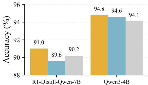
GSM8K
