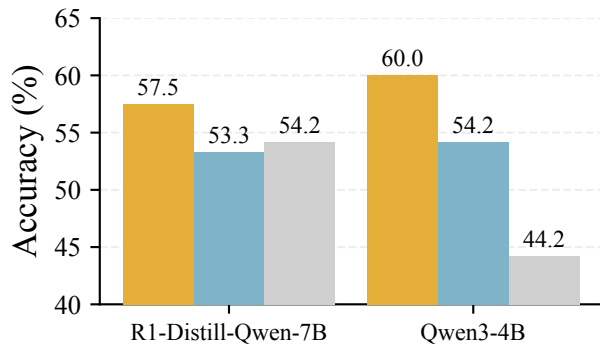
AIME24
