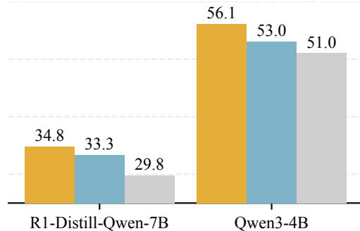
GPQA-D
