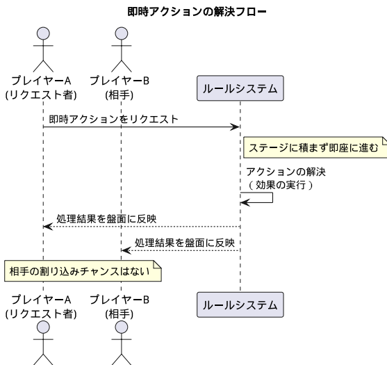
Fig. 5.5 即時アクションの解決フロー
