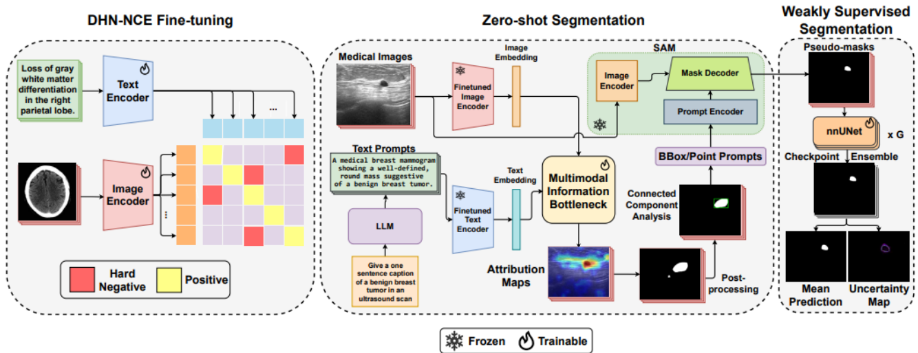
Hình 4. Sơ đồ kiến trúc luồng dữ liệu từ embedding đa phương thức, saliency map M2IB và sinh segmentation mask bằng SAM [1].
