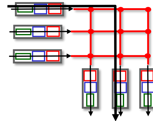
3x3 crossbar
